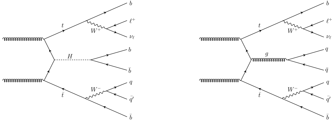
Figure 0.1.: Diagrammes de Feynman des processus (gauche) t\bar{t}H(H \rightarrow b\bar{b}) et (droite) t\bar{t} + \text{jets} .
