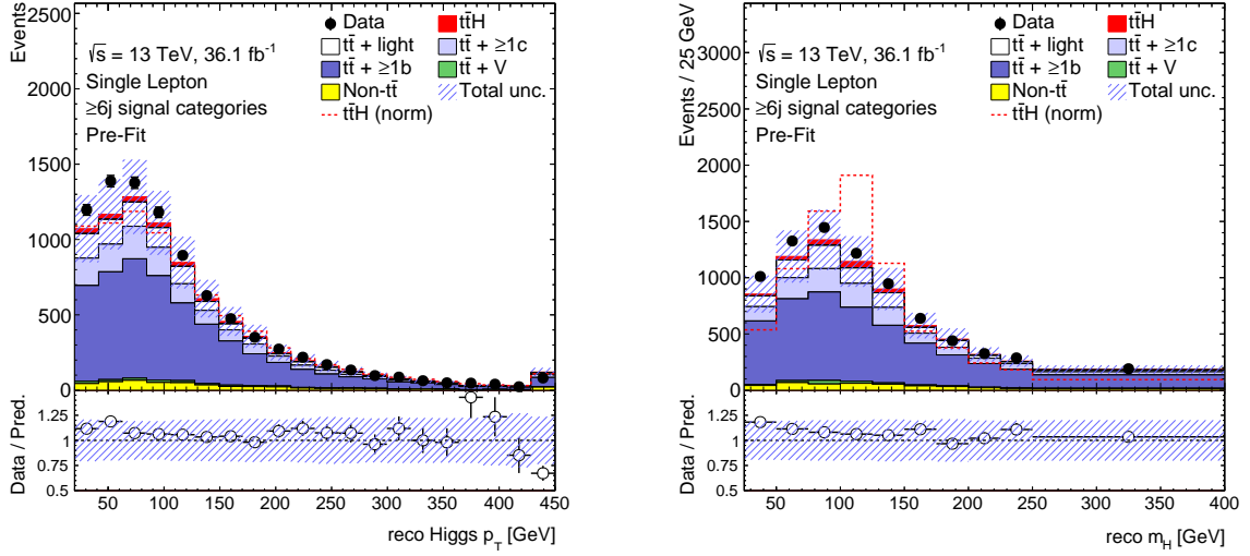
Figure 0.5.: Comparaison des distributions prédites et observées dans les données pour (gauche) le p_T et (droite) la masse du candidat au boson de Higgs. Seuls les événements satisfaisants les selections pour les régions de signal sont gardés. La zone hachurée représente l'incertitude prédite totale (systematique et statistique) sans prendre en compte les incertitudes de normalisation des composantes t\bar{t} + \geq 1b et t\bar{t} + \geq 1c . Les prédictions sont montrées avant les corrections apportées par l'ajustement.
