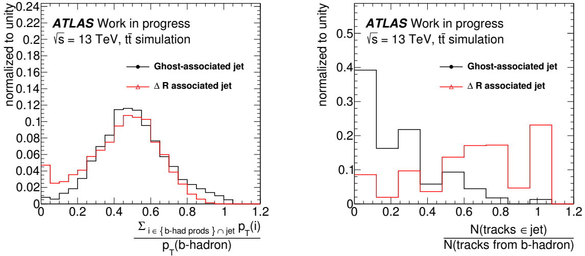
Figure 0.3.: Distributions de la fragmentation d'un hadron b en deux jets, l'un des deux jets étant étiqueté b par association \Delta R (le \Delta R -associated-truth-jet) et l'autre par association fantôme (ghost-associated-truth-jet). (Gauche) fraction d'énergie du b -hadron retrouvé dans chacun des deux jets. (Droite) nombre de traces issues du hadron b retrouvé dans chaque jets divisé par le nombre total de traces issues du hadron b .
