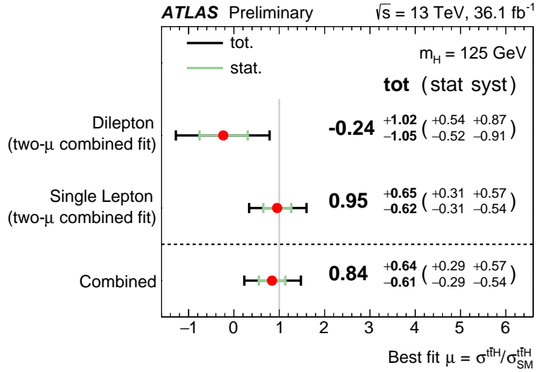
Figure 0.7.: Valeurs de \mu pour les canaux un-lepton, deux-lepton et leur combinaison, observées après l'ajustement statistique des deux canaux combinés aux données.
