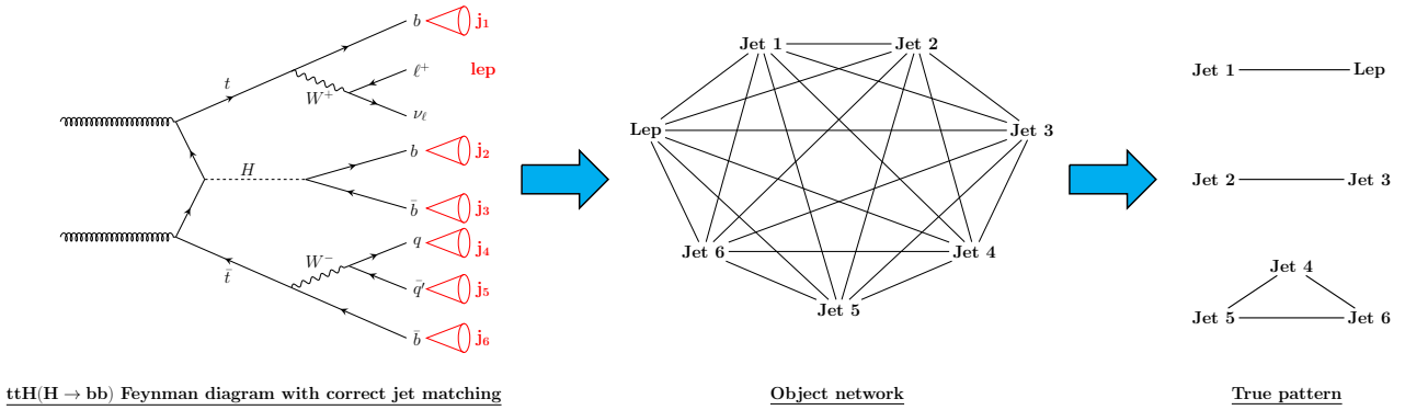
Figure 0.6.: Schéma de la reconstruction sur réseau. (Gauche) Diagramme de Feynman avec les jets associés à chaque parton. (Milieu) diagramme formé par les objets reconstruits. (Droite) Motif original recherché par les algorithmes d'agglomération et de résolution sur le réseau.
