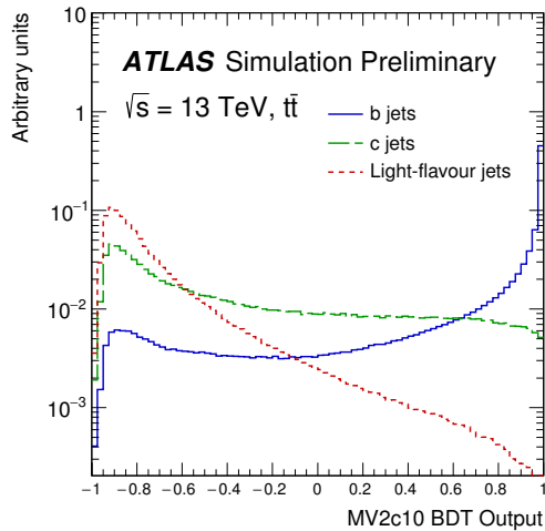
Figure 0.2.: (Gauche) Schéma représentant un b -jets accompagné de deux light -jets. (Droite) Discriminant final du b -tagging, MV2, pour la différentiation des b -jets contre les c -jets et light -jets.
