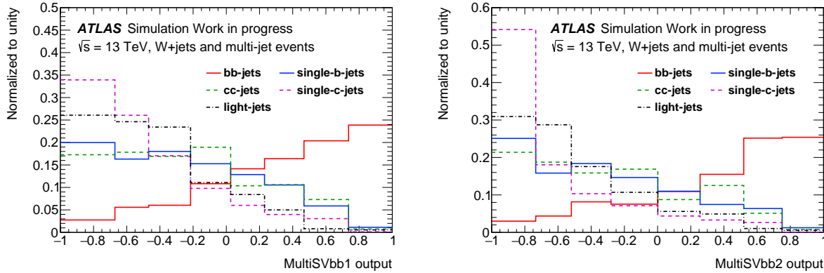
Figure 0.4.: Distributions de sortie des BDTs pour les algorithmes (gauche) MultiSVbb1 et (droite) MultiSVbb2 pour chaque saveur de jet.
