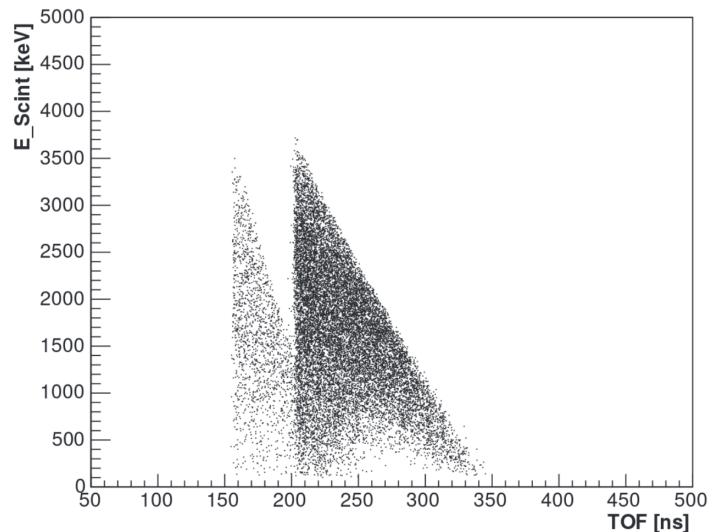
(b) CENPA spectra (Feb. 2015 data) [CENP15].
