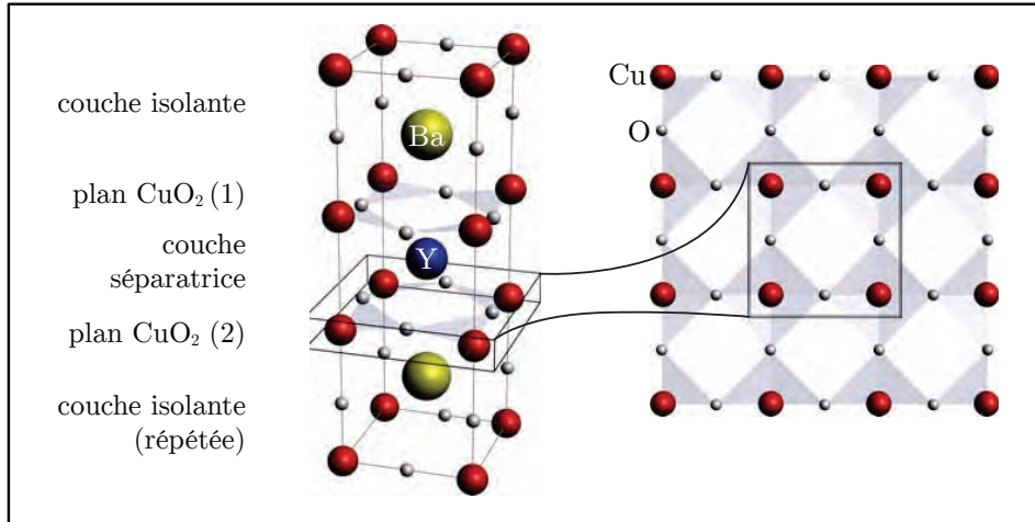
Figure 1 : Structure cristallographique typique des cuprates supraconducteurs. Le matériau considéré est précisément \text{YBa}_2\text{Cu}_3\text{O}_7 , dont la maille élémentaire contient deux plans \text{CuO}_2 séparés par une couche d'Yttrium. Les paires de plans sont séparées par du Barium, de l'oxygène et des chaînes \text{CuO} .
