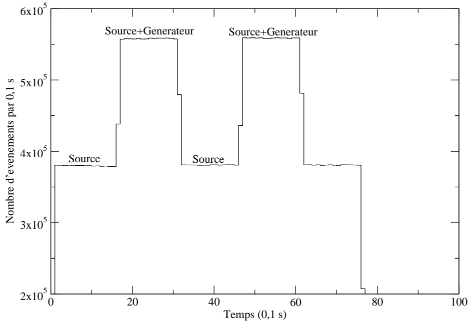
FIG. 2.5 – Nombre d'événements enregistrés avec une source radioactive puis avec une source et un générateur d'impulsions au cours d'une mesure du temps mort fixe de l'acquisition.
