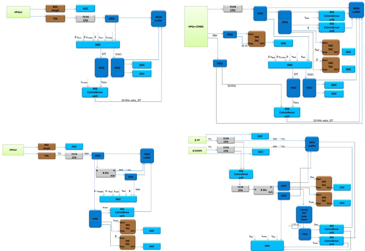
FIG. 4.5 – Schémas de l’électronique d’acquisition des données de l’expérience E622S pour l’étude de la décroissance de ^{18}\text{Ne} . Ils décrivent de haut en bas et de la gauche vers la droite le traitement des signaux électroniques issus du détecteur HPGe1 situé au niveau de la chambre de collection du faisceau, les détecteurs HPGe CENBG et HPGe2 situés en regard de la chambre basse de mesure de la décroissance de l’activité collectée et des deux photomultiplicateurs associés au détecteur plastique (voir la figure 4.4).
