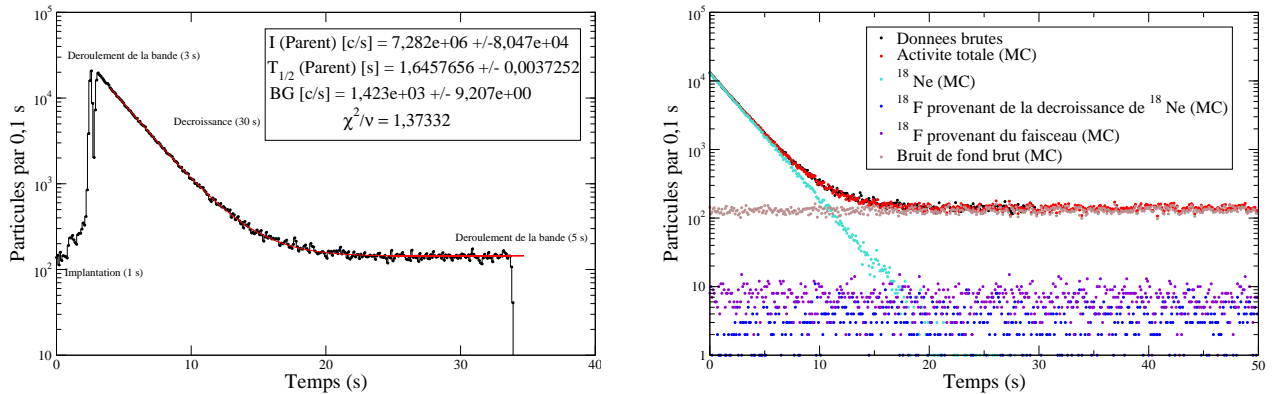
FIG. 4.11 – Le graphe de gauche présente le spectre en temps des particules \beta détectées lors de la mesure la plus longue de la durée de vie de ^{18}\text{Ne} . Les données brutes sont présentés en noir et le meilleur ajustement en rouge. Le graphe de droite montre à l’aide d’un calcul Monte-Carlo (MC) les différentes composantes de l’activité obtenues à partir de l’ajustement. L’activité de ^{18}\text{Ne} est présentée en bleu clair, celle du ^{18}\text{F} provenant du faisceau en violet, celle du ^{18}\text{F} provenant de la décroissance de ^{18}\text{Ne} en bleu foncé et celle du bruit de fond ambiant en marron.
