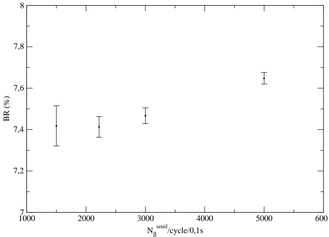
FIG. 4.25 – Valeurs moyennes obtenues pour les différents seuils appliqués à l’analyse des rapports d’embranchements des mesures individuelles représentées dans la figure 4.24.
