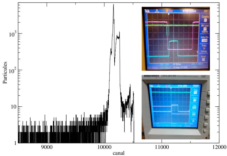
FIG. 4.19 – La figure représente pour une mesure caractéristique du rapport d'embranchement de la décroissance super-permise de ^{18}\text{Ne} , le spectre d'empilement obtenu au moyen d'un module TAC à partir du signal d'empilement généré par l'amplificateur associé au détecteur HPGe CENBG. Les photographies insérées dans le spectre montrent deux exemples des signaux envoyés par le module TAC au codeur ADC : dans la photographie du haut, le signal d'empilement en bleu arrive au début de la porte de codage de l'ADC visible en rose. Dans la photographie du bas, le signal issu du module TAC arrive au tout début de la porte de codage.
