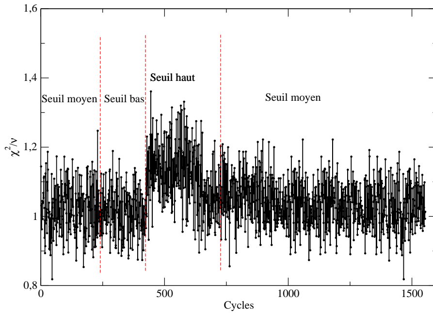
FIG. 2.14 – La distribution du paramètre \chi^2 normalisé en fonction des cycles enregistrés avec le premier détecteur pour les trois seuils de discriminateur (bas, moyen et haut).
