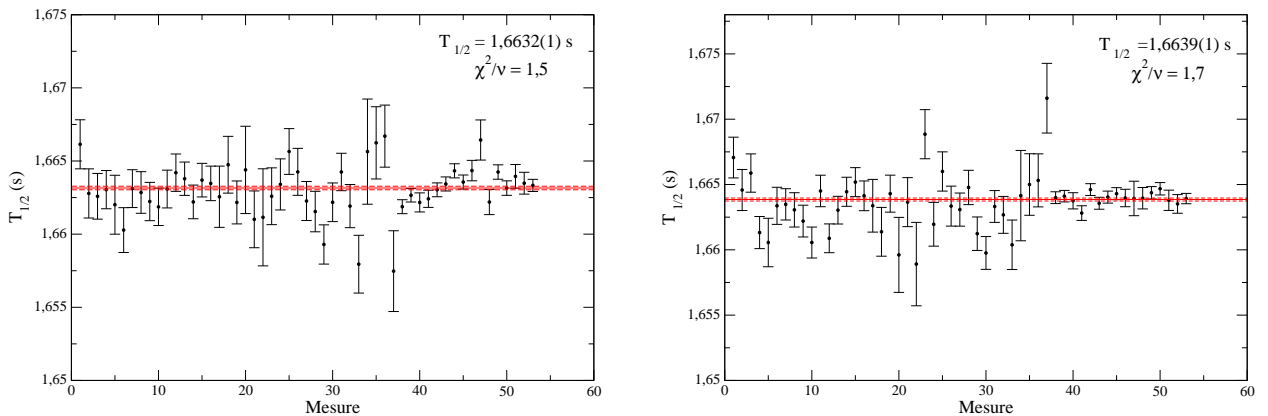
FIG. 2.15 – Temps de vie de ^{18}\text{Ne} extrait des 53 mesures effectuées avec le premier détecteur (à gauche) et le deuxième détecteur (à droite) de l'ensemble SCEPTAR. Les lignes rouges continues et en pointillés représentent la valeur moyenne des 53 mesures et l'incertitude statistique sur cette valeur.
