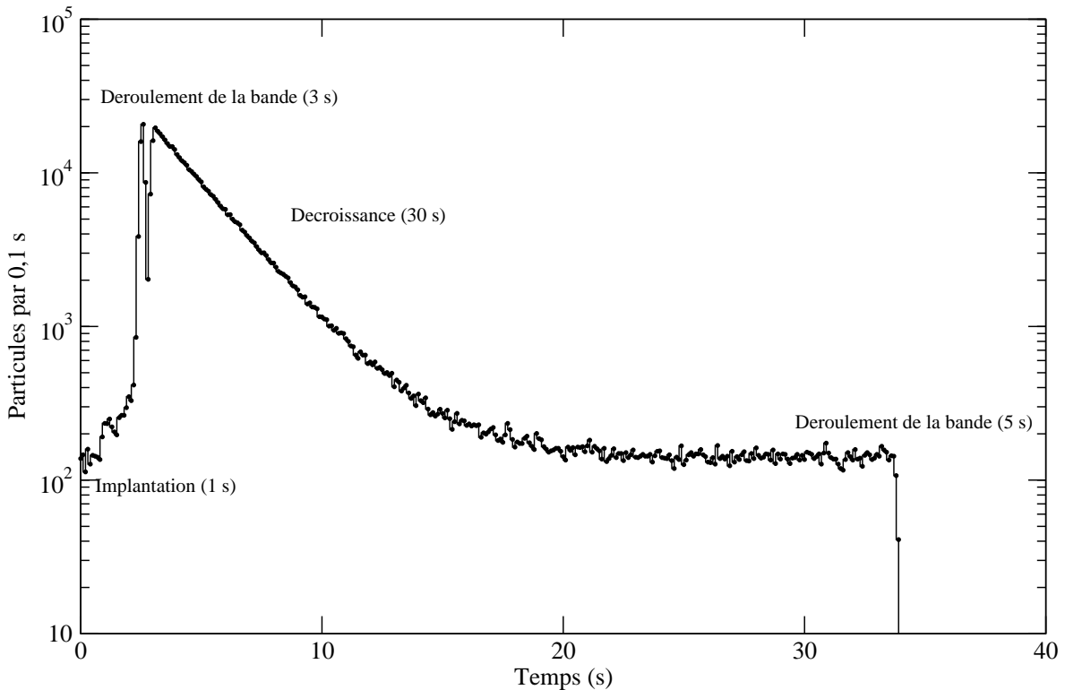
FIG. 4.6 – Spectre en temps des évènements de décroissance \beta observés à l'aide du détecteur plastique lors d'une mesure représentative de la durée de vie de ^{18}\text{Ne} . Les différentes phases des cycles de mesure sont indiquées.
