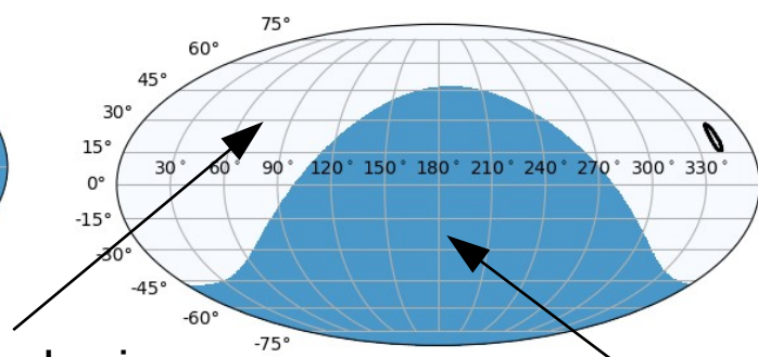
GW170818
