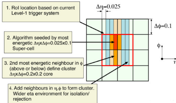
FIG. 2: Calcul de la forme de la gerbe au niveau 1, basé sur l'usage de clusters formés dans la deuxième couche du calorimètre à partir d'une granularité améliorée ( \Delta\eta \times \Delta\phi = 0.025 \times 0.1 ) de la région d'intérêt
