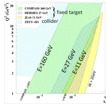
FIGURE 5: Domaine cinématique en x_{bj} et Q^2 couvert par les différentes expériences étudiant le DVCS.
