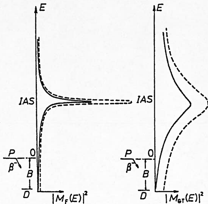
Fig. 57 : Formes des résonances isobariques analogue et de Gamov-Teller calculées par la théorie globale ([TAK72]).
