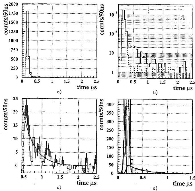
Figure 4.21 Sélections des gammas de l'isomère 734 keV à partir des spectres temps des Ge: a)b) Spectre gamma prompt(pointillé) et isomère(noir), c) Fit de la différence,d)En noir les événements déterminés comme expliqué dans le texte.
