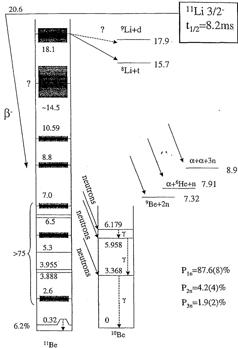
Figure 3.1 Schéma partiel de décroissance du ^{11}\text{Li} indiquant les seuils pour les nombreux canaux ouverts. Les valeurs de P_n sont de [Bor97]
