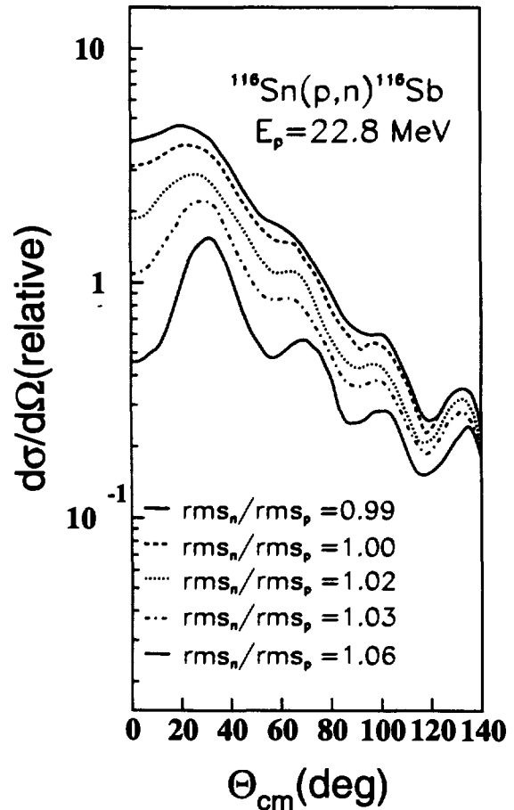
Figure 1.5: Distributions angulaires pour la réaction ^{116}\text{Sn}(p,n)^{116}\text{Sb} [Sch76].
